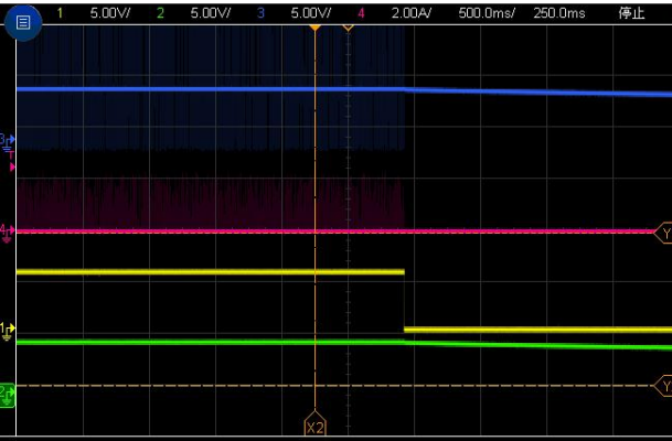
CH1: EN CH2:VOUT CH3:SW CH4:IL
