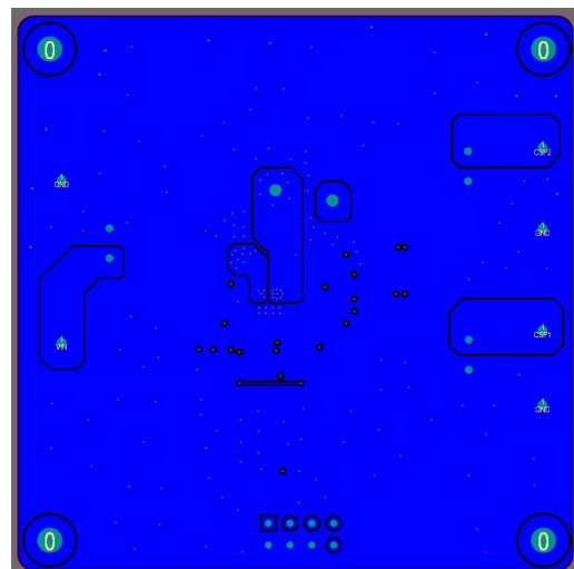
Fig. 11.2-3 Bottom Layer
