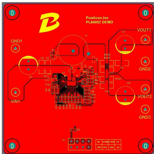
Fig. 11.2-2 Top Layer
