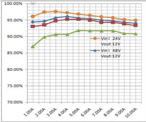
Fig. 3 效率曲线
