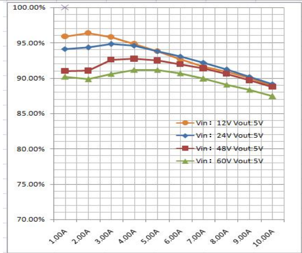
Fig. 4 效率曲线
