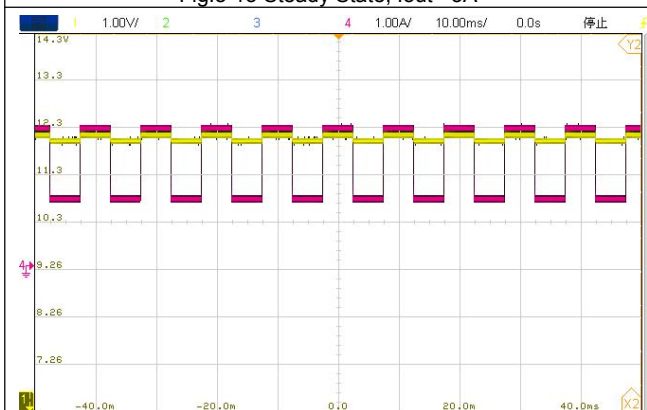
CH1:VOUT CH4:IL
