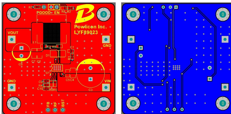
Fig. 11-2-3 PCB
