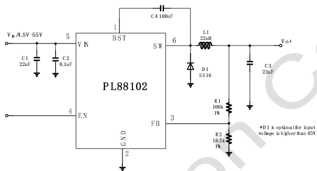
Fig. 1 Schematic
